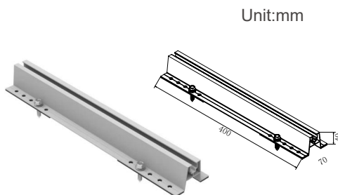
• WQ-IRM-40 H40 IR \pi Mini Rail
