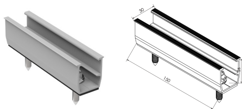
WQ-TRU-30 H30 TR U Mini Rail
