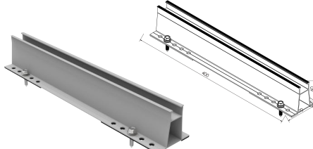
WQ-TRΠ-60 H60 TR π Mini Rail
