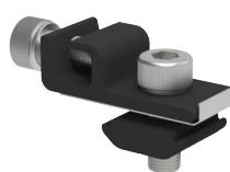
WQ-TR-GL-B Black TR Grounding Lug
