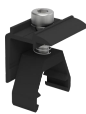
• WQ-CRE-3035-B Black CR End Clamp
